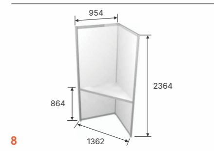
8 Kampinė lentyna Corner shelf 29 €
